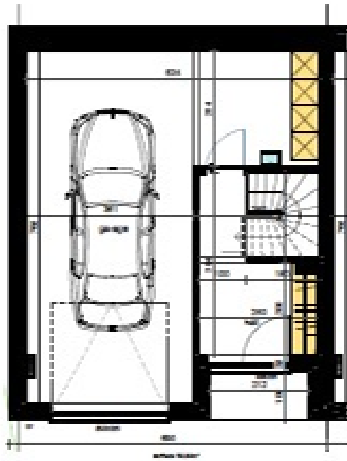
sous-sol 1:100
